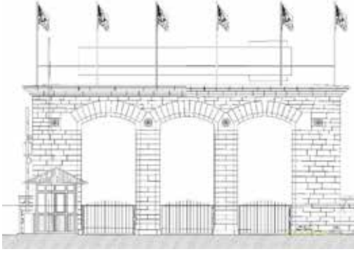
Stad giriş kapısının güney cephesinin çizimi (E. Z. TOMAR)
